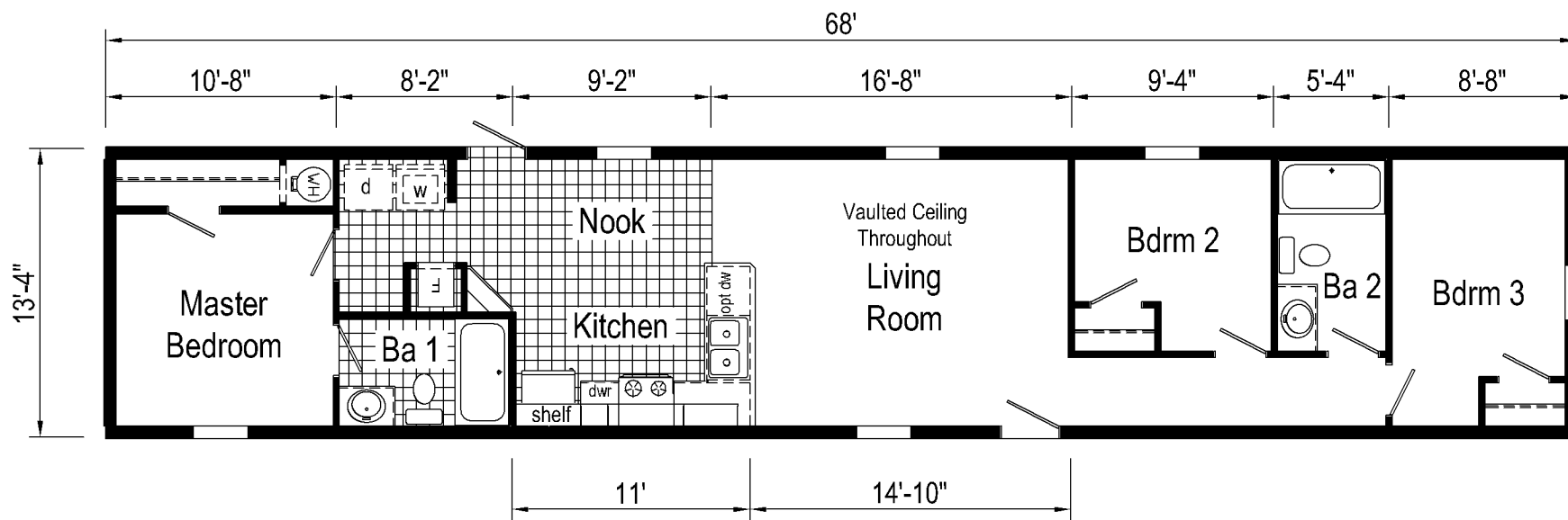
DS102-A 1468 Approx . 907 Sq. Ft.
